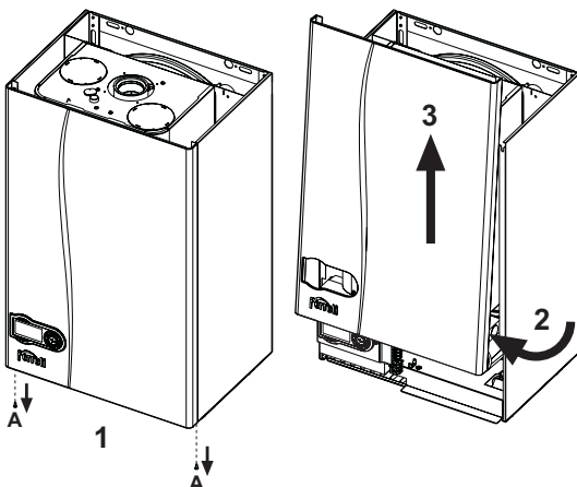
fig. 28 - Apertura de la carcasa
