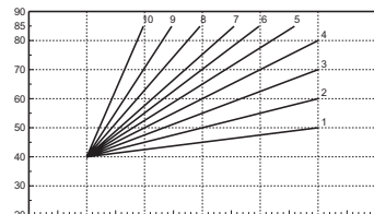
fig. 15 - Esempio di spostamento parallelo delle curve di compensazione
