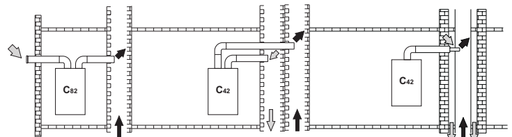
рис. 25 - Примеры подсоединения к дымоходам (⇨ = Воздух / ⇨ = Продукты сгорания)
