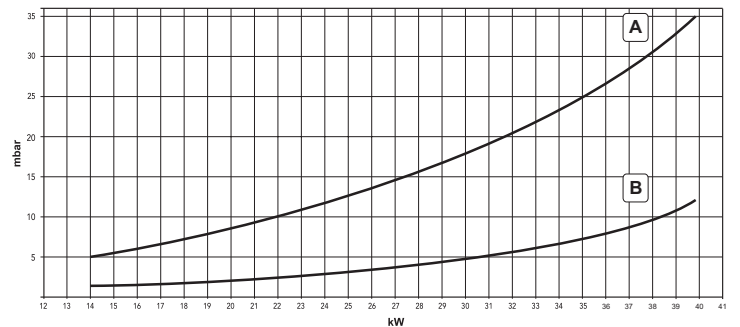
fig. 37 - Diagrama presión / potencia DIVAtop MICRO F 37
