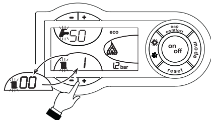
fig. 26 - Modalidad TEST (potencia de la calefacción = 100%)
