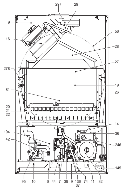
fig. 32 - Vue générale DIVAtop MICRO F 37
