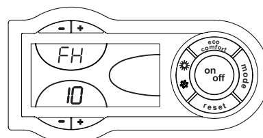
fig. 6 - Accensione caldaia
