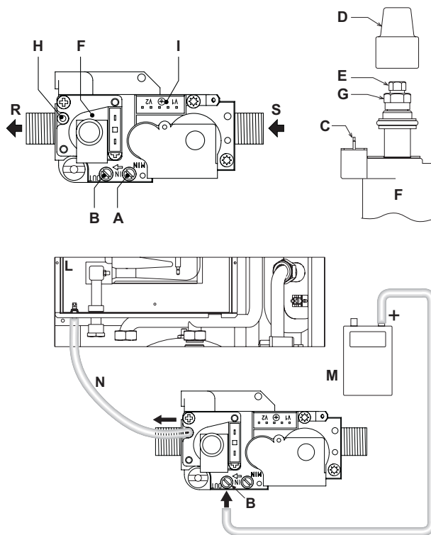
рис. 27 - Газовый клапан
