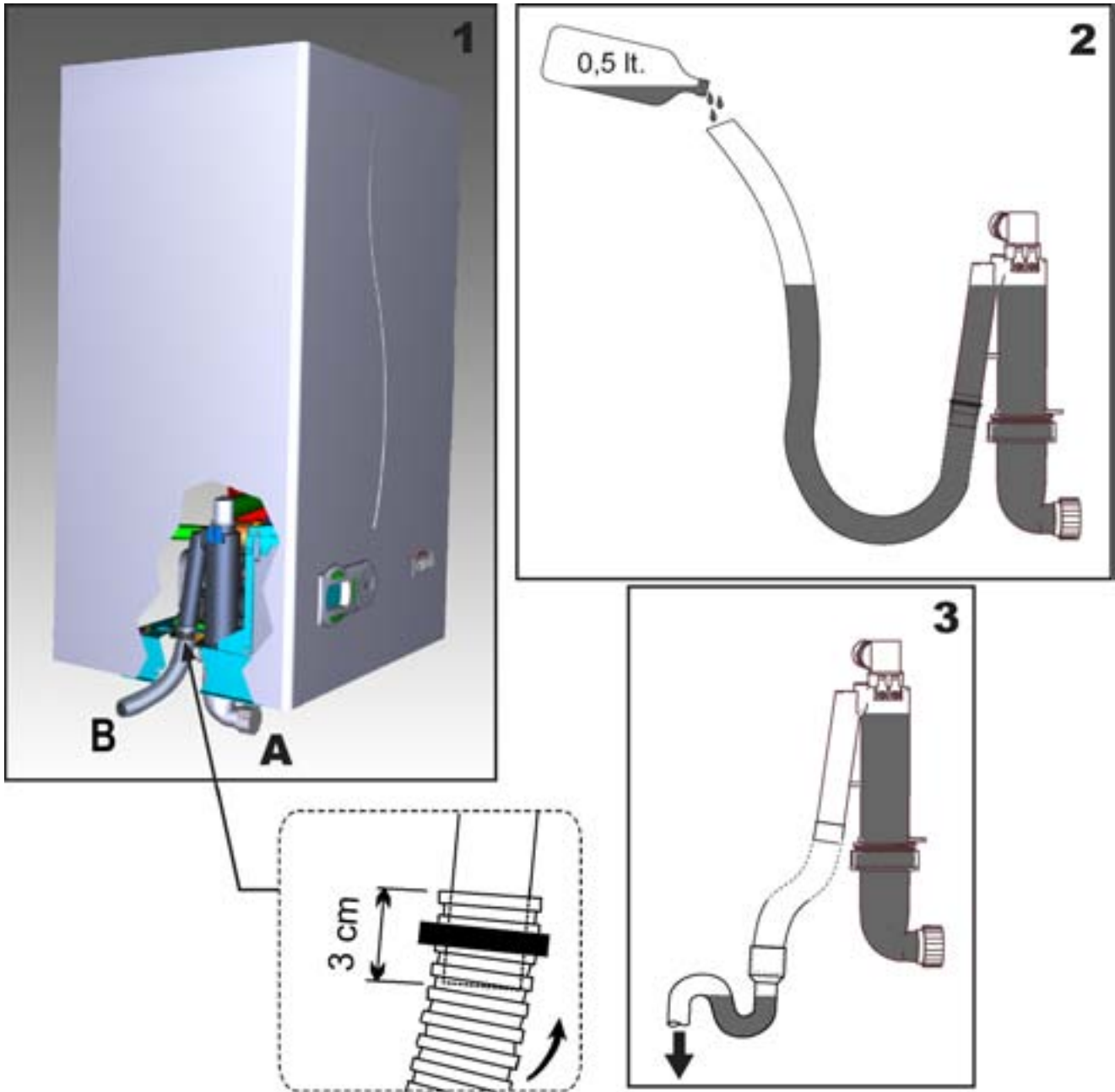
рис. 26 - Крепление трубы для слива конденсата
