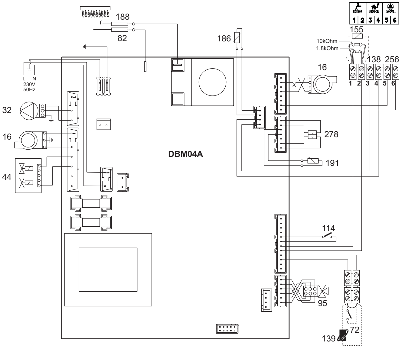
рис. 34 - Электрическая схема
