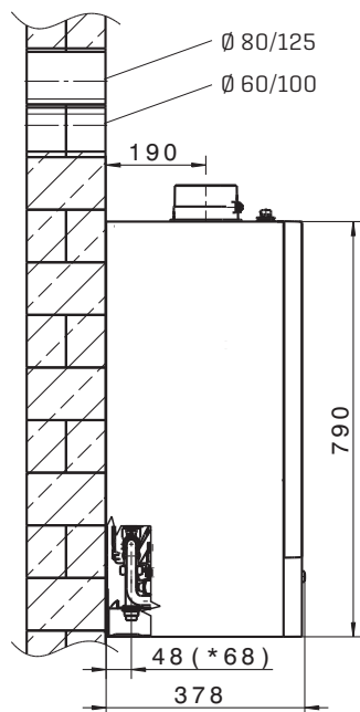
Вид сбоку
