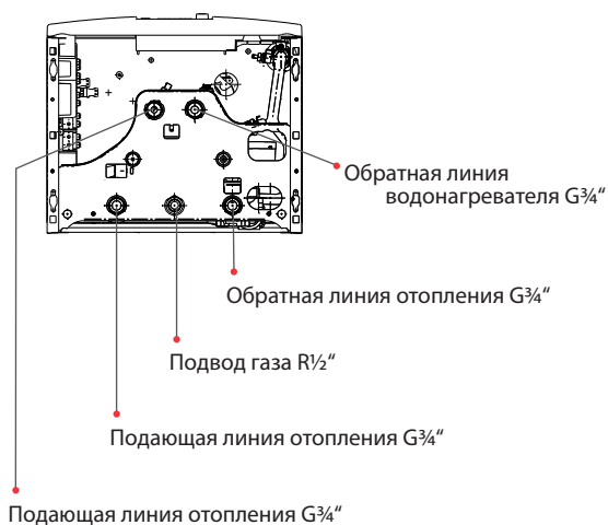
Вид спереди
