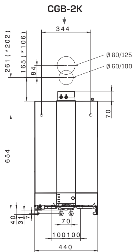
Вид спереди
